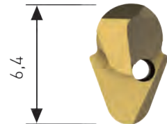
Größe 4 (HWS = 105124) Size 4
