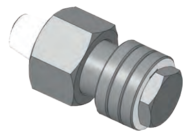
Spannmutter clamping nut FDM 1736B (M=M24x1) o. FDM 1736C (M=M25x1,75)
