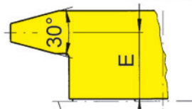
Profil frontal du porte outils Profilo frontale del portainserito
