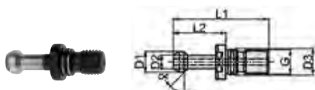
Tiranti AZB MAS/BT 45° (JIS B 6339) con foro interno
