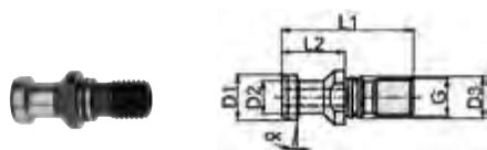
Tiranti AZB ISO 7388/II-B con foro interno
