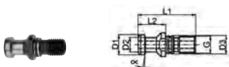
Tiranti AZB DIN69872-A con foro interno
