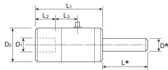
Portautensili rotanti attacco cilindrico
