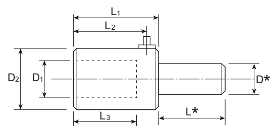
Portautensili non rotanti
